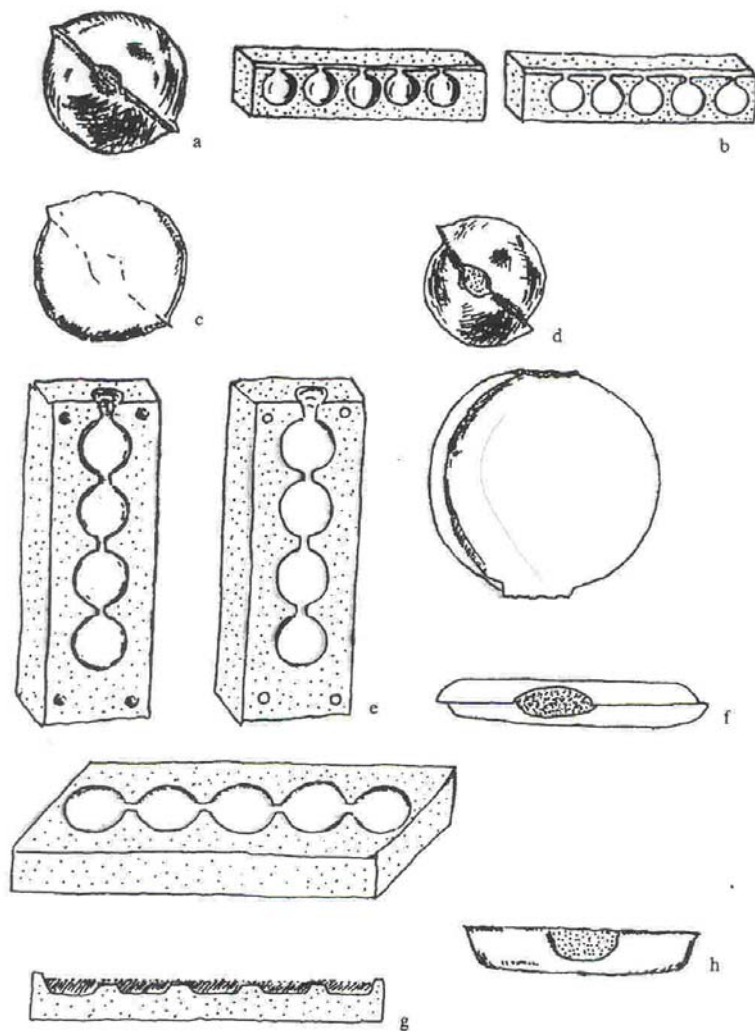
LÁMINA IV a) Flan globular. b) Formas múltiples. c) Flan globular aplastado antes de la acuñación. d) Flan globular obtenido con valvas no bien yuxtapuestas. e) Molde cerrado para flanes de disco, aplastados o lenticulares. f) Flan de disco y punto de fractura. g) Molde abierto. h) Flan obtenido en molde abierto y punto de fractura. Según A. Finetti.
